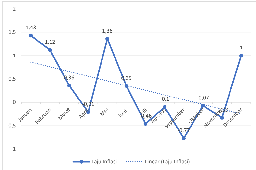
Gambar 2 - 10 Tingkat Inflasi Regional Kab. Majene Tahun 2021
